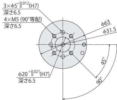
R軸 (M4:手首旋回) の取付面 [単位:mm]
