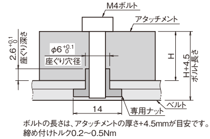
アタッチメント取付部詳細
