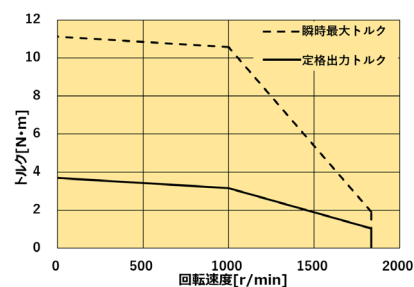
減速比 7
