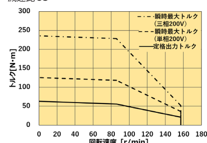
減速比 35
