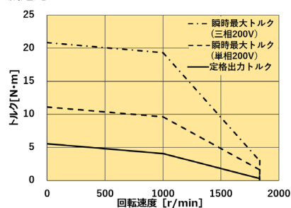
減速比 7
