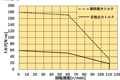
減速比 50
