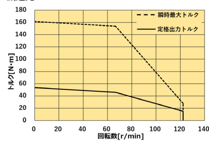
減速比 45
