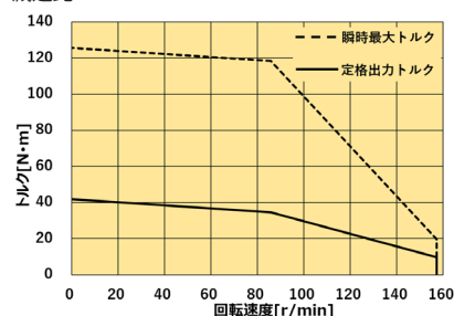
減速比 35
