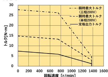
減速比 4
