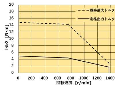
減速比 4
