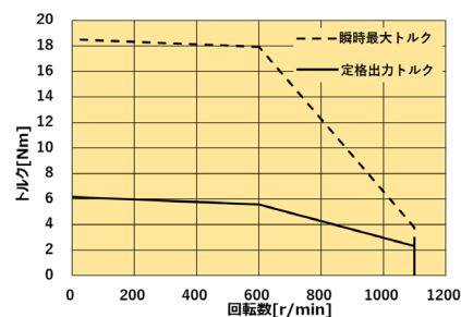
減速比 5
