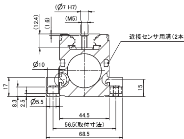
【B-B 断面】
