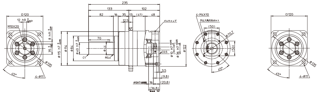
軸出力 (キータップ付き)
