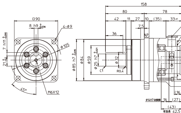
軸出力 (キータップ付き)
