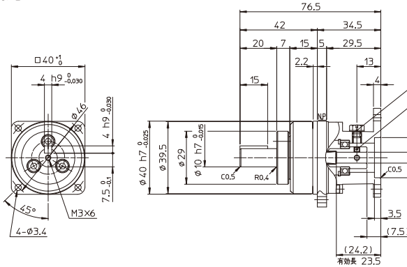
軸出力 (キータップ付き)
