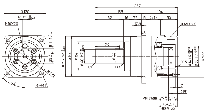
軸出力 (キータップ付き)
