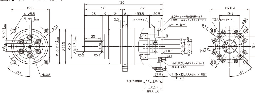
(キーなしタップなし)
