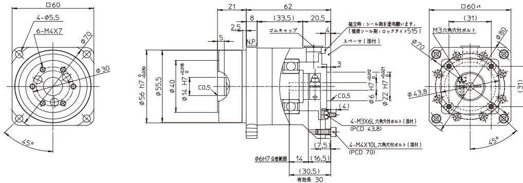
軸出力 (キータップ付き)
