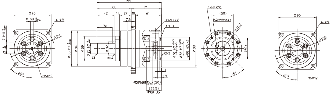
軸出力 (キータップ付き)
