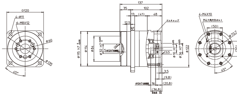
軸出力 (キータップ付き)
