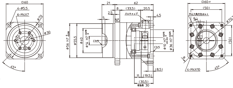
軸出力 (キータップ付き)
