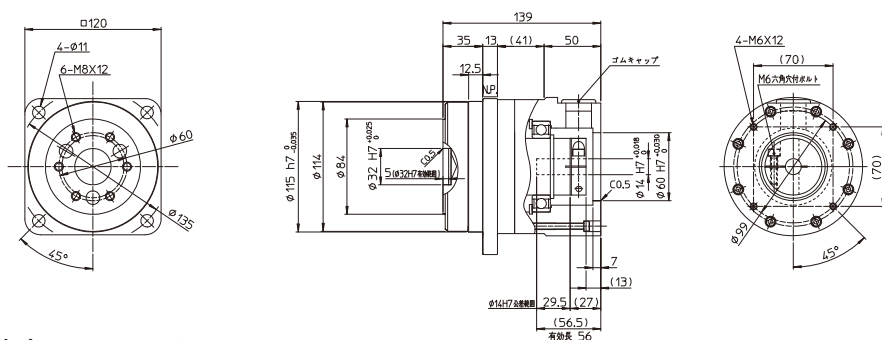
軸出力 (キータップ付き)
